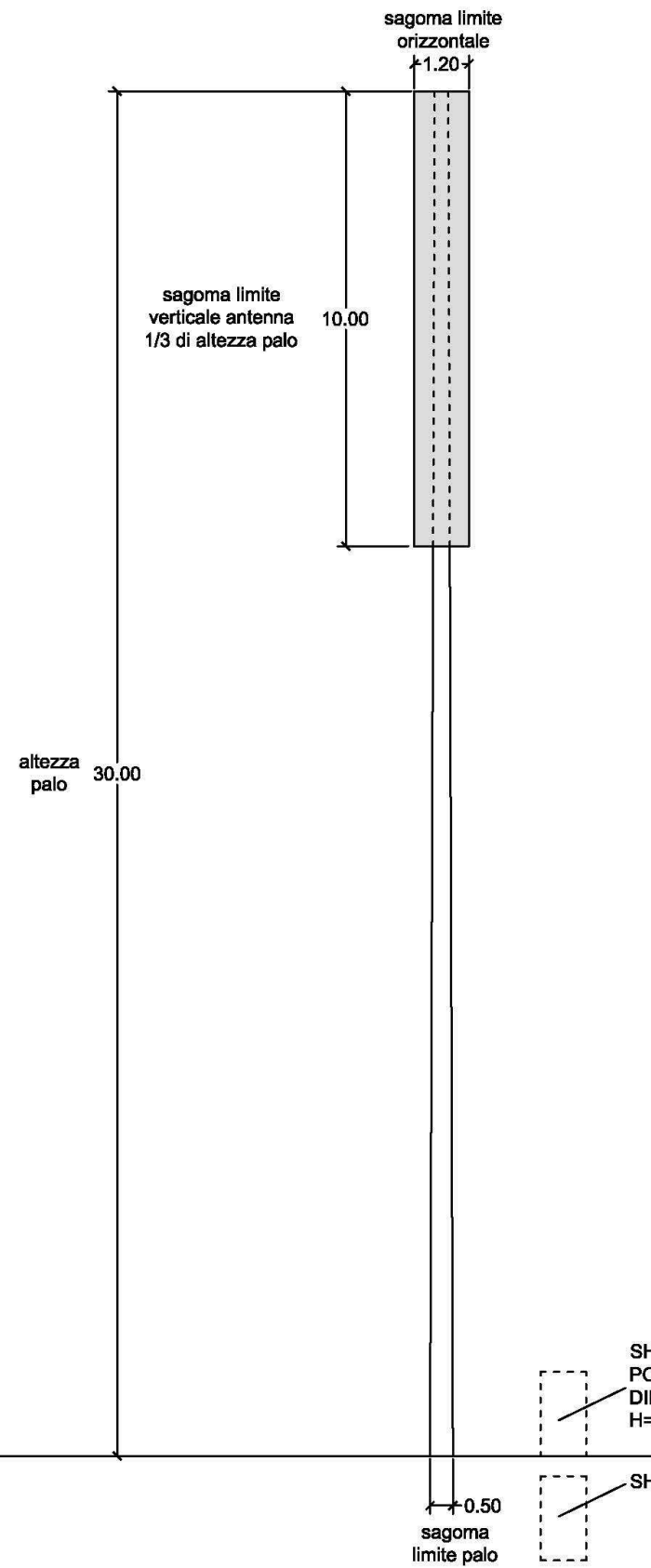
STRUTTURA IN PALO RASTREMATO CON PANNELLO CILINDRICO CHE SCHERMA ALLA VISTA LE ANTENNE
